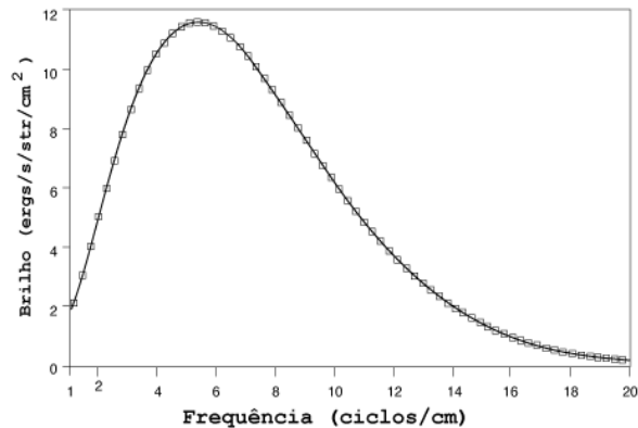
Figura 27.07: Resultados do satélite COBE, mostrando que a radiação do fundo do Universo segue mesmo a lei da radiação de Planck.
