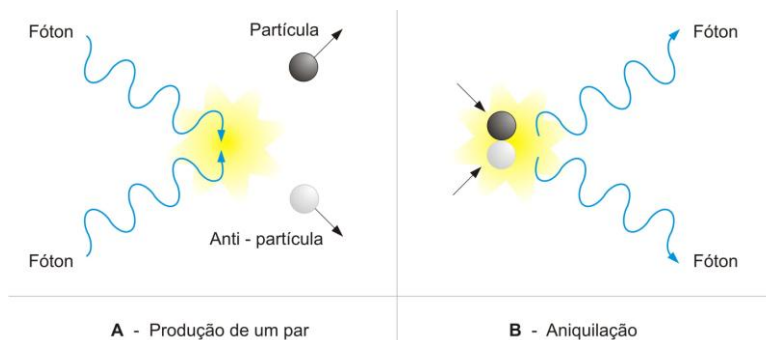
Figura 27.04: À esquerda dois fótons se aniquilam produzindo partículas e antipartículas, logo a seguir, à direita, as partículas e anti-partículas se aniquilam e se convertem em fótons novamente.
