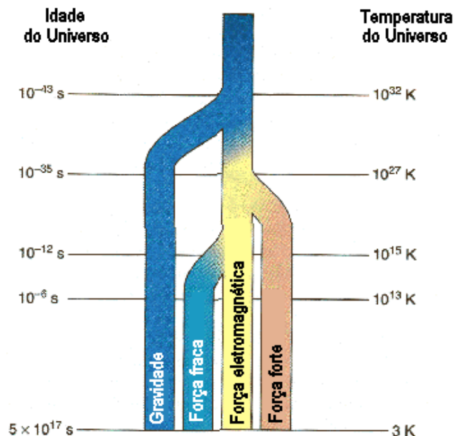
Figura 27.03: Gráfico ilustrando as épocas em que ocorreram as separações das quatro forças da natureza, as quais encontravam-se unificadas na era de Planck.
