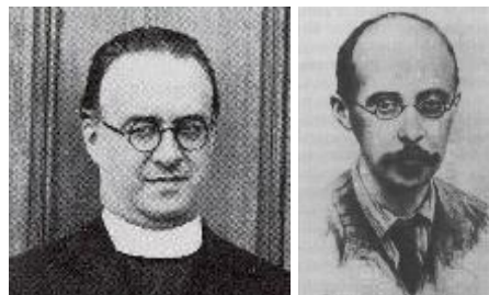
Figura 27.02: À esquerda Georges Lemaître (1894-1966), à direita Alexander Friedmann (1888-1925).
