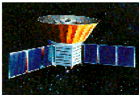
Figura 27.06: Satélite COBE.
