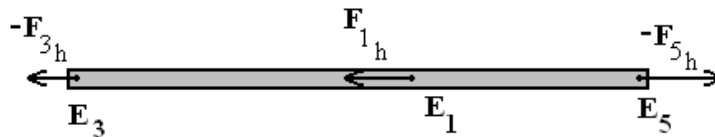
Figura 6 – Forças horizontais exercidas sobre o travessão superior da balança.
