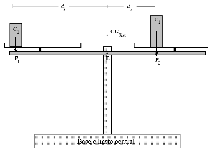
Figura 2- Uma “balança impossível”.
