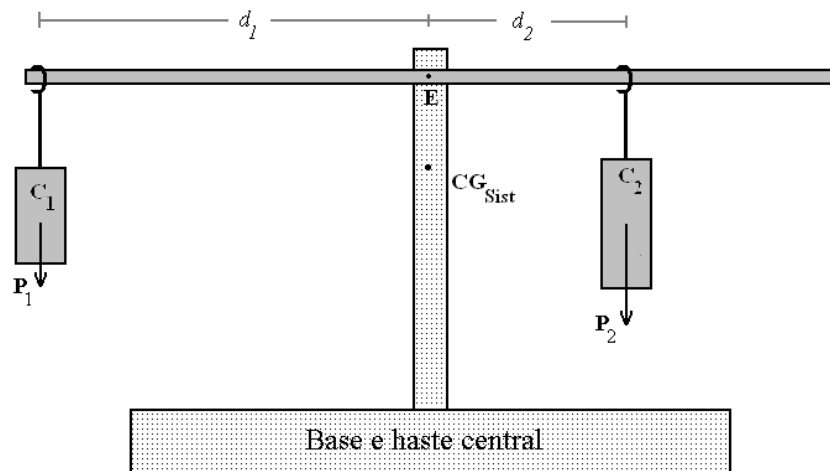
Figura 1- Esquema simplificado de uma balança.
