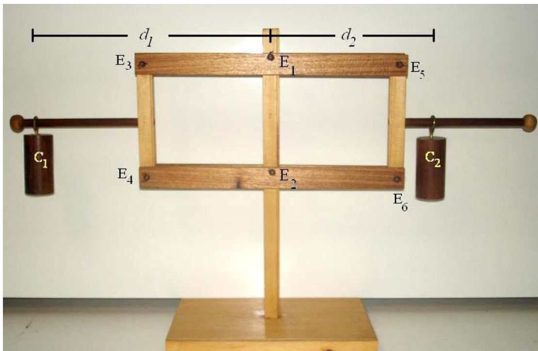
Figura 3 – Balança de Roberval simétrica equilibrando dois corpos de mesmo peso posicionados a distâncias diferentes em relação aos eixos fixos de rotação E_1 e E_2 .
