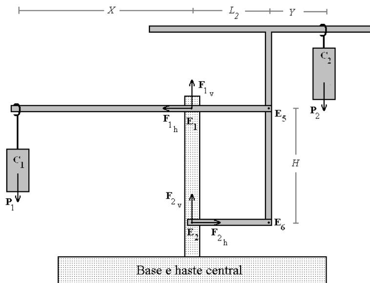
Figura 7 – A semi-balança de Roberval.
