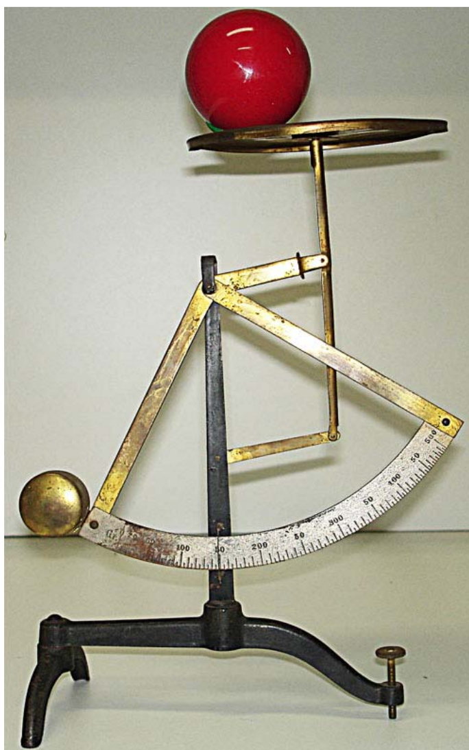
Figura 14 – A balança postal incorpora o mecanismo de Roberval para servir de apoio ao prato de pesagem. Leitura: 150 g.
