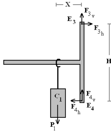
Figura 5 – Forças exercidas sobre a peça lateral esquerda da balança.
