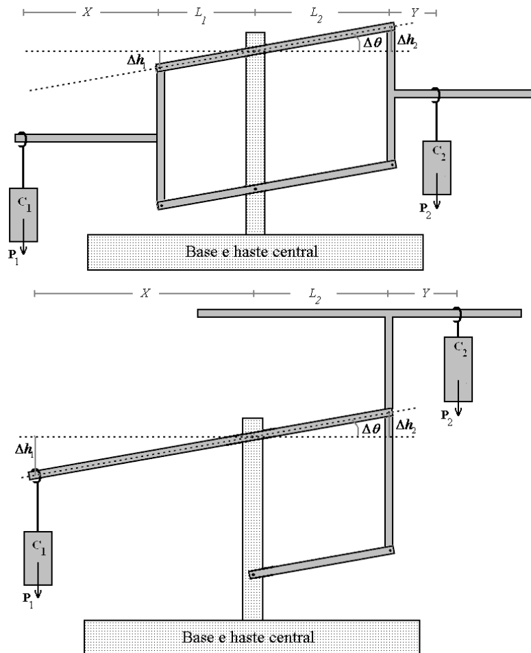
Figura 9 – Balanças deslocadas da posição de equilíbrio.
