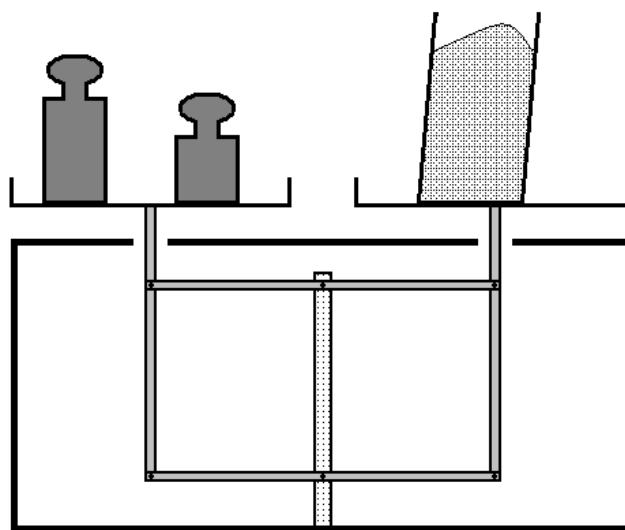
Figura 12 – Representação esquemática de uma balança de Roberval comercial.
