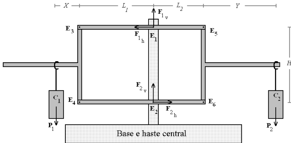
Figura 4 – Balança de Roberval assimétrica
