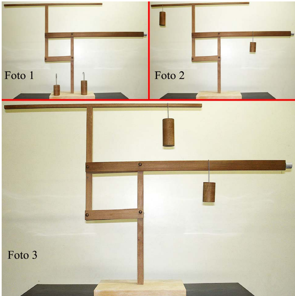
Figura 10 – Comportamento inusitado para a semi-balança de Roberval.
