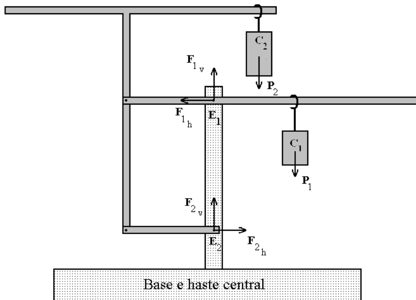
Figura 11 – Torques das forças exercidas pelos eixos anulam os torques dos pesos.
