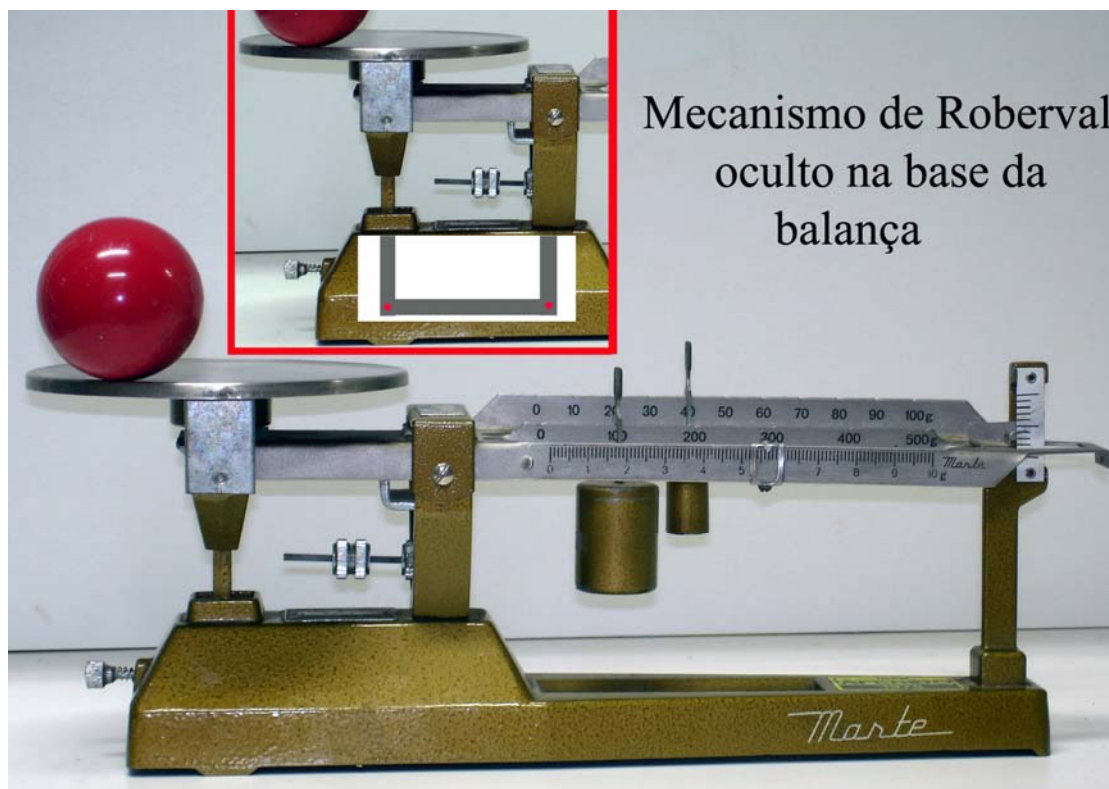
Figura 13 – Balança utilizada em laboratórios didáticos. Leitura: 145, 7 g.
