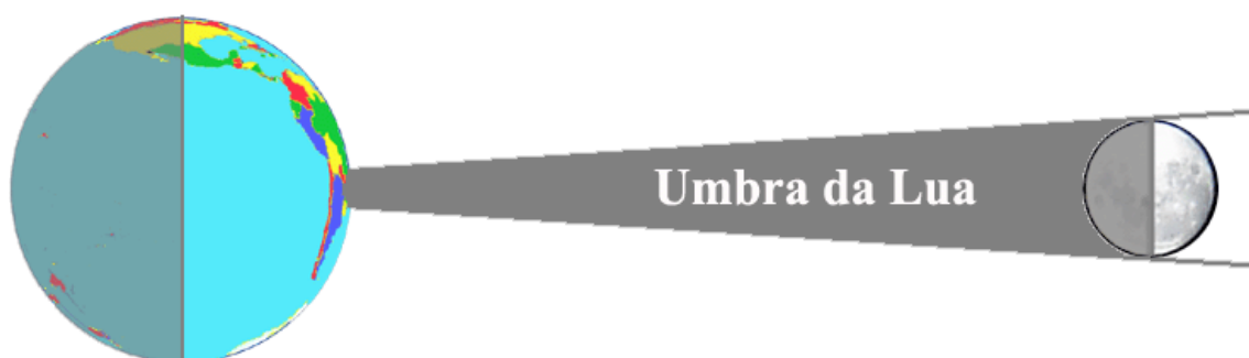
Figura 11 – O vértice do cone de sombra ou umbra da Lua se encontra sempre próximo à superfície da Terra durante um eclipse solar total, determinando que o diâmetro da sombra da Lua na Terra seja muito menor do que o diâmetro lunar.
