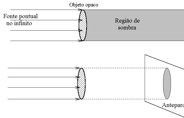
Figura 4. Para uma fonte pontual no infinito: região de sombra e a sombra sobre um anteparo. O tamanho da sombra não varia com a distância entre o objeto opaco e o anteparo.
