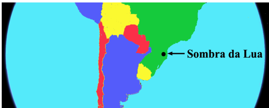
Figura 12 – A sombra da Lua na superfície da Terra durante um eclipse solar total tem um diâmetro com no máximo cerca de 250 km. Somente observadores dentro dessa sombra “encolhida” poderão perceber o eclipse como total.
