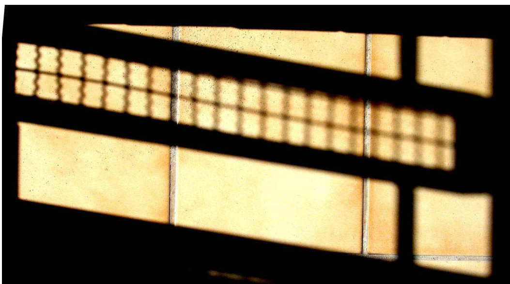
Figura 10 – Grade de arame intercepta a luz solar produzindo sombra e penumbra.
