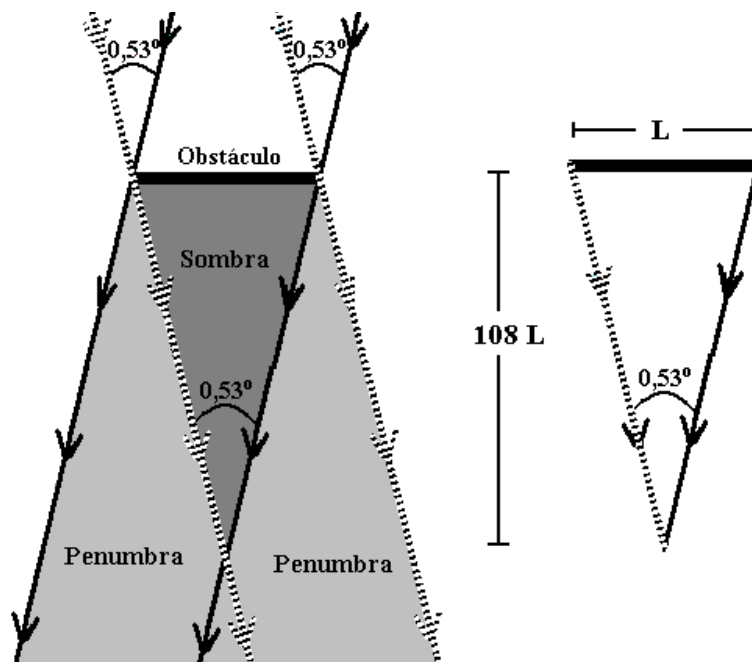
Figura 9 – Representação esquemática da região de sombra produzida por um obstáculo que impede a passagem dos raios luminosos solares.
