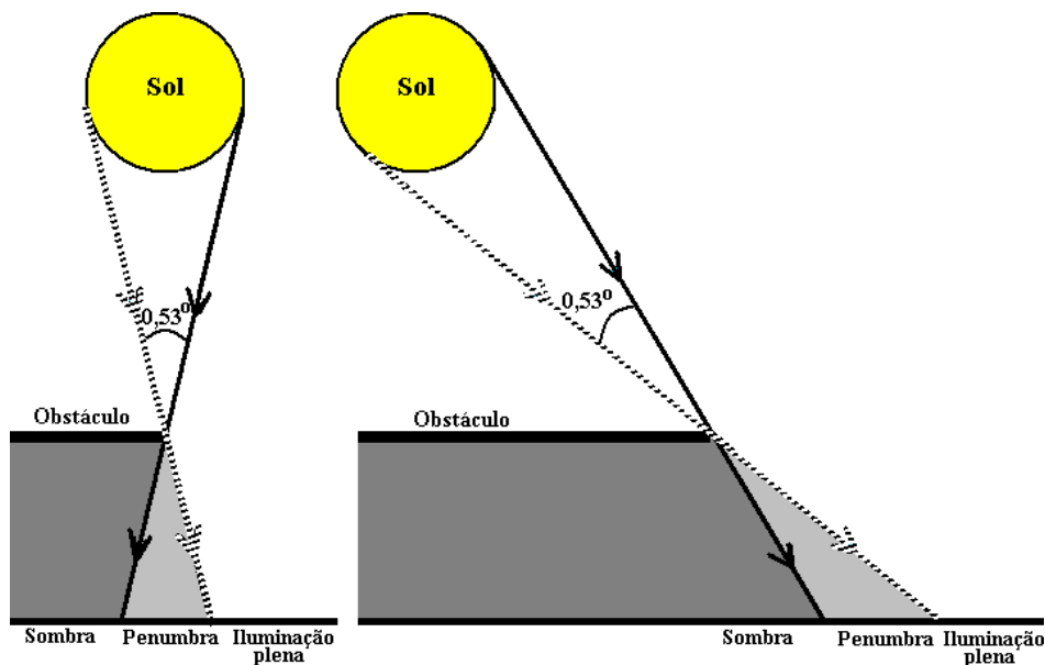
Figura 8 – A luz solar que se origina em regiões diferentes do disco solar produz sombras com bordas não definidas, contornadas por uma região de penumbra.
