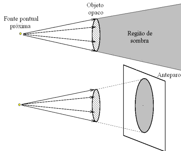
Figura 3. Sombra produzida por uma fonte pontual próxima: a região de sombra e a sua seção transversal, como aparece ao incidir a luz da fonte em um anteparo. A sombra é tanto maior quanto mais distante do anteparo estiver o objeto opaco, e quanto mais próxima deste se encontrar a fonte.
