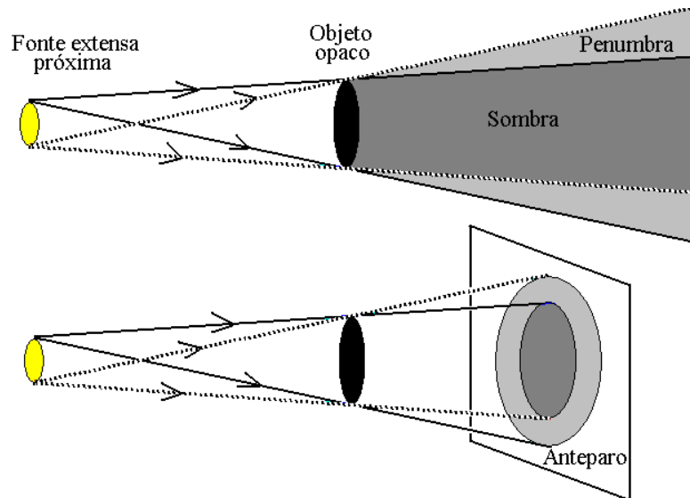
Figura 6. Sombra produzida por uma fonte extensa próxima e menor do que o objeto opaco que intercepta seus raios luminosos. A região de sombra é dominante sobre a região de penumbra, de forma que as bordas da sombra ficam mais nítidas. Essa nitidez é tanto maior quanto menor for a fonte.
