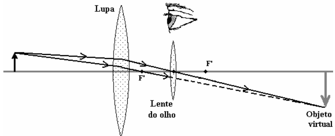
Figura 4 – A imagem real conjugada pela lupa é um objeto virtual para a lente do olho.
