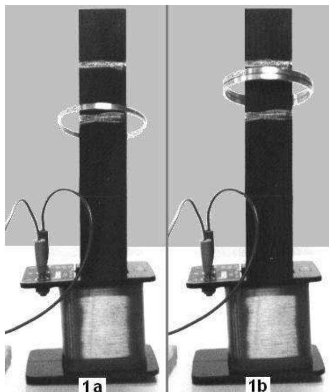
Figura 1 – Demonstração da “levitação magnética” com uma argola (1a) e duas argolas (1b).
