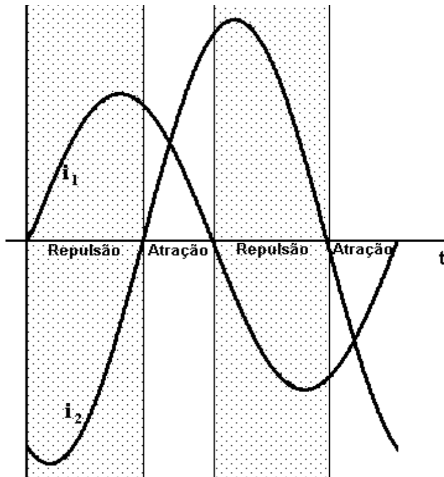
Figura 6 – Correntes elétricas na bobina e no anel defasadas por mais do que \frac{1}{4} ciclo e menos do que \frac{1}{2} ciclo.
