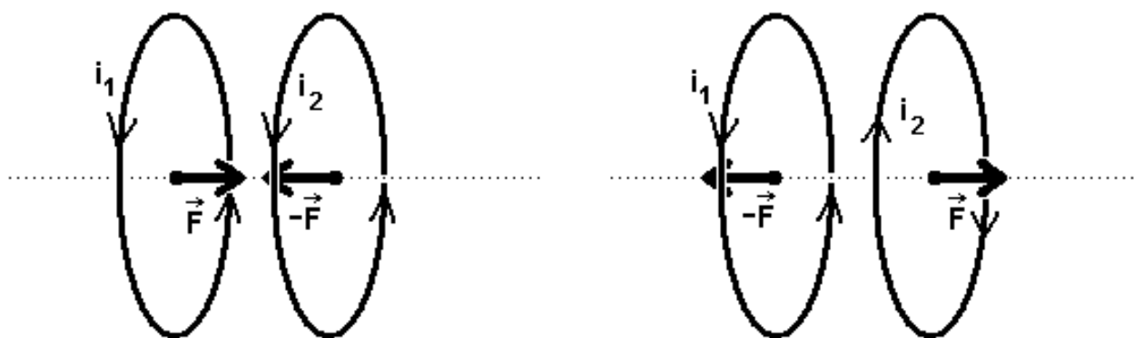
Figura 2 – Duas espiras com corrente elétrica interagem magneticamente.
